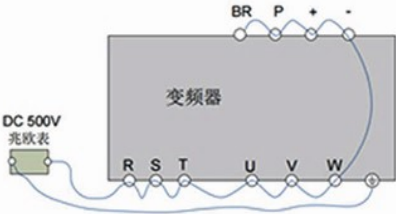
图 8-1 主回路绝缘测试示意图
