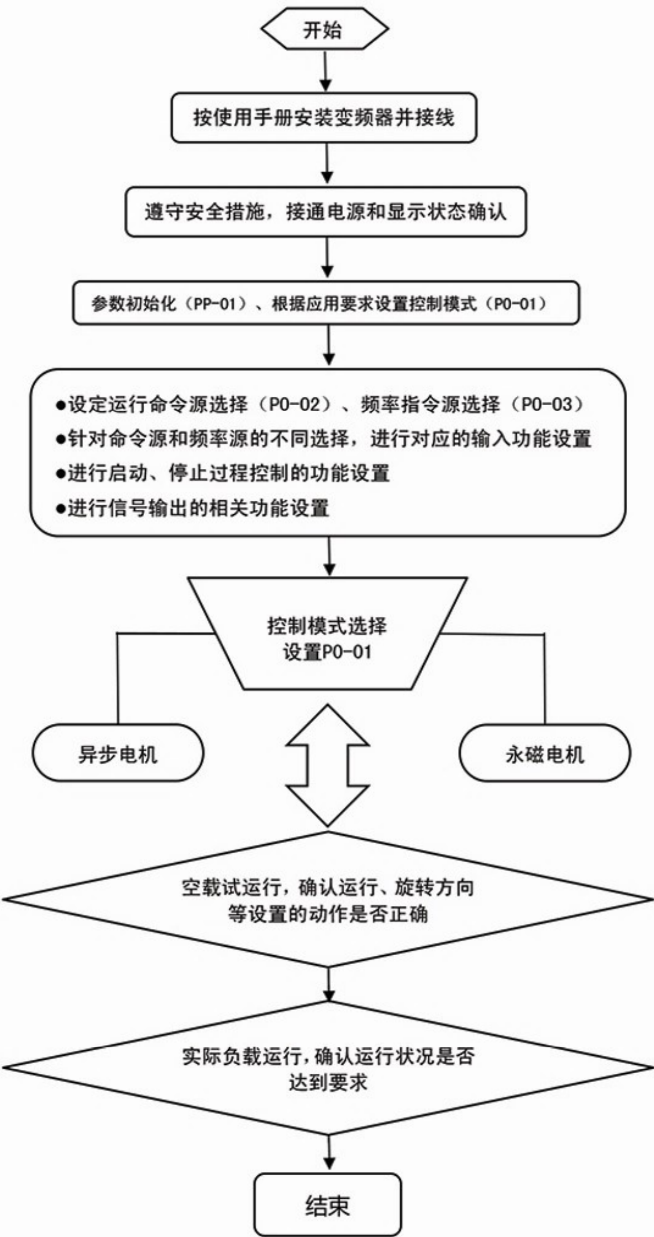
图 3-2 变频器调试总流程图
