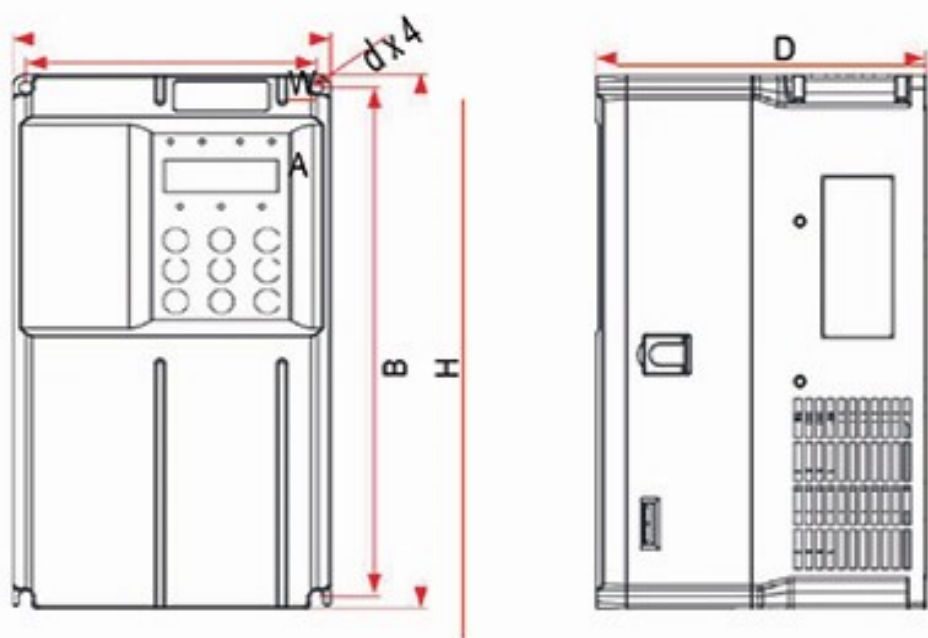
图 1-1 EST900-T0.4GB ~ EST900-T15GB 外型尺寸及安装尺寸示意图
