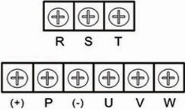
图 3-28 EST900-030G4 ~ EST900-045G4 主回路端子分布图
