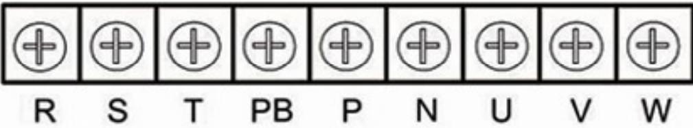
图 3-28 EST900-030G4 ~ EST900-045G4 主回路端子分布图
