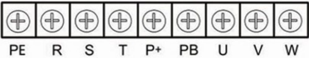
图 3-27 EST900-R75G4 ~ EST900-4 R0G4 主回路端子分布图
