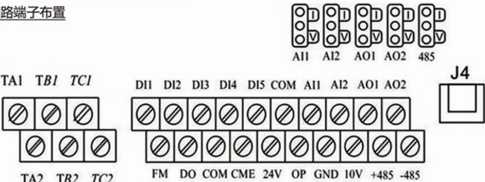
图 1-5 控制回路端子布置图
